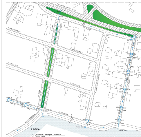
Planta de Drenagem - Trecho B Escala: 1/1000
