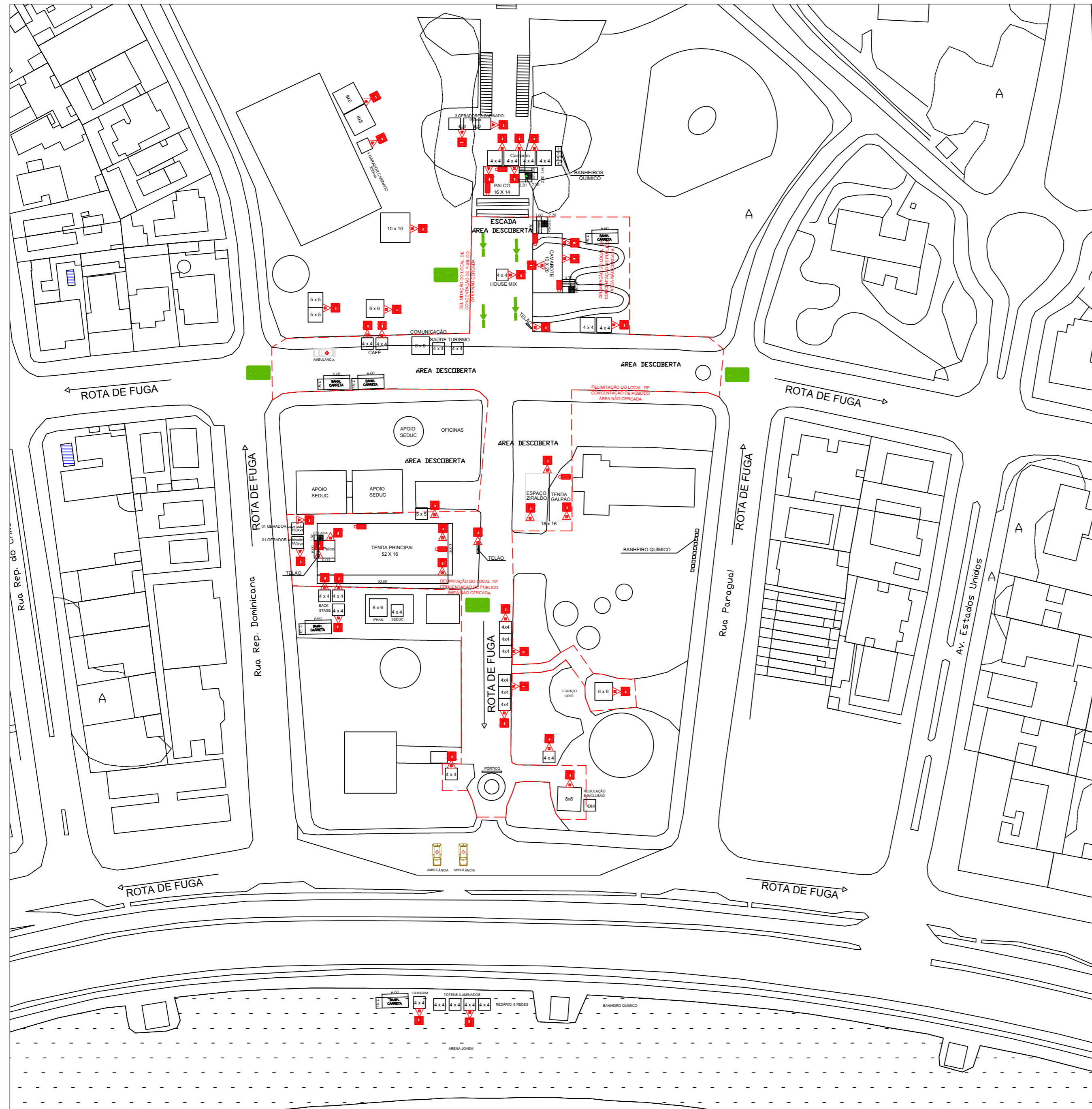
1 PLANTA BAIXA ESC: 1/1000
